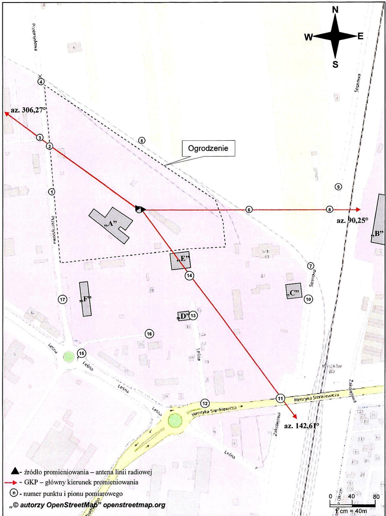
Rys. 1. Usytuowanie punktów i pionów pomiarowych w otoczeniu instalacji radiokomunikacyjnej Stacja Netia WYSWB006-WYSWM00002 Wyszaków, ul. Przemysłowa 4
